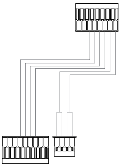
UniDrone E900 双云台吊舱线 UniDrone E900 Dual Gimbal Pod Cable
